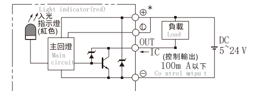
感应器连接图 < 原点及端点 >
